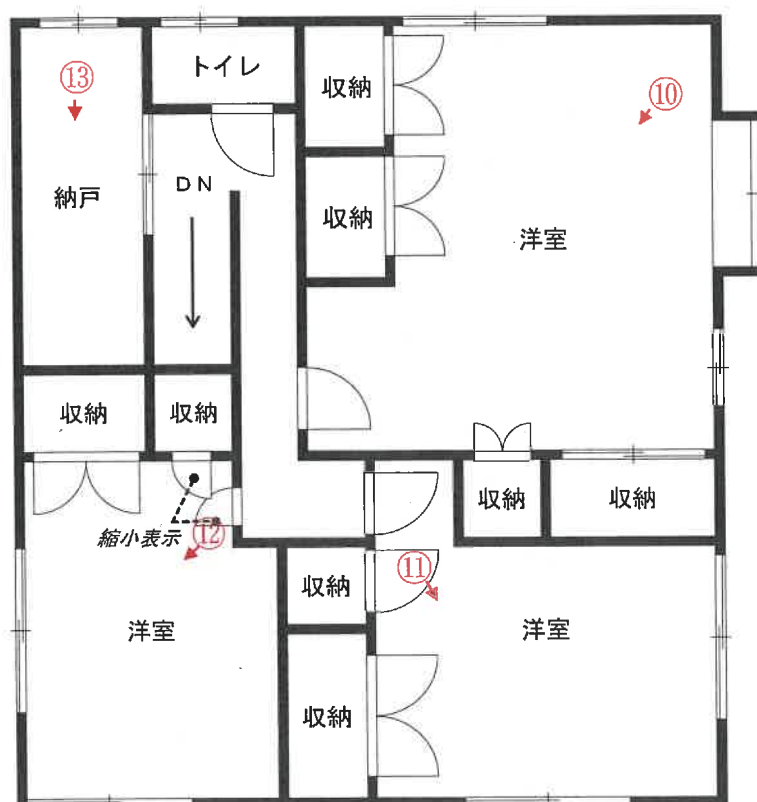
2階平面図
