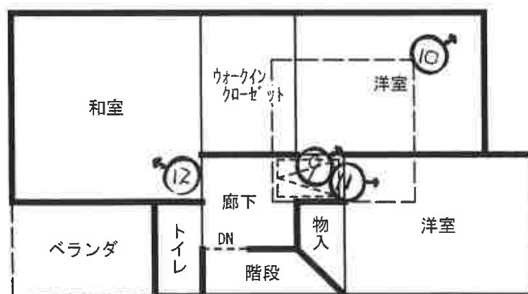
2階平面図
