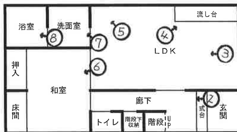
1階平面図
