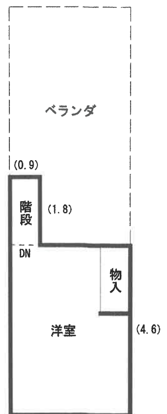
3階平面図 (現況床面積 約 16.4㎡)
