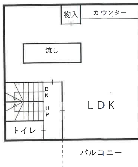
2階
