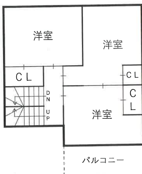
3階
