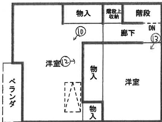
3階平面図
