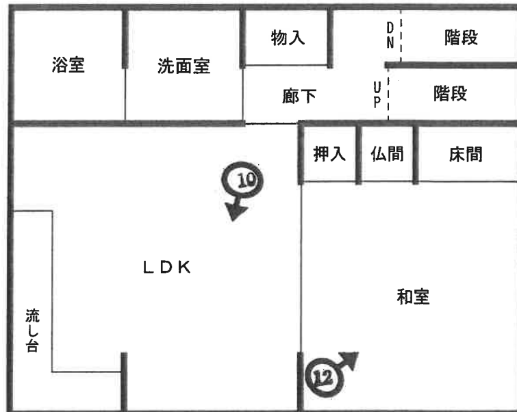
2階平面図
