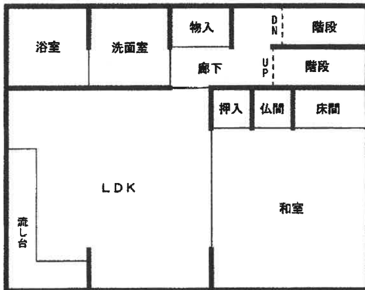
2階平面図
