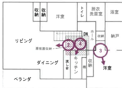
<2階>
