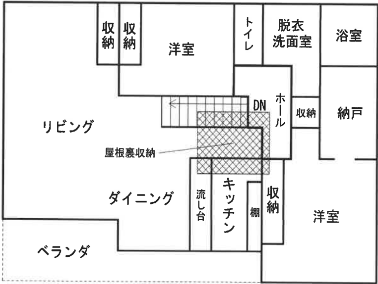
< 2階 >
