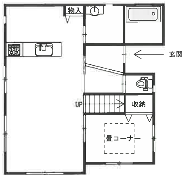
1 階平面図
